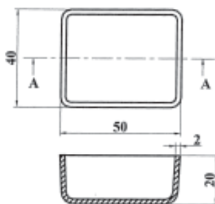
Sec A-A
